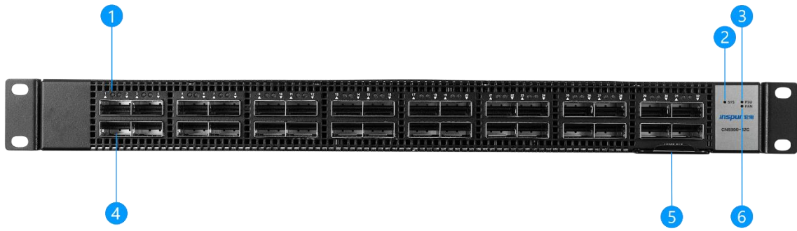
图 1-1 CN9300-32C 前面板示意图
