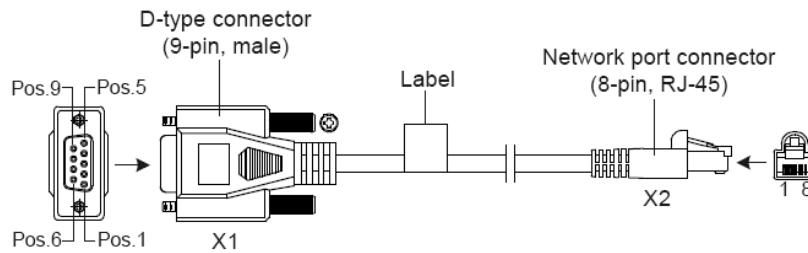
图 1-3 DB9 to RJ45 控制台接口连接线缆
