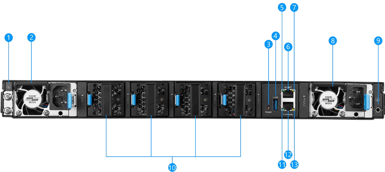
图 1-2 CN9300-32 后面板示意图
