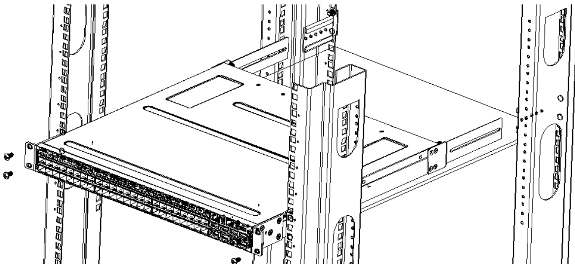
图 2-2 交换机安装至机架（带托盘）示意图
